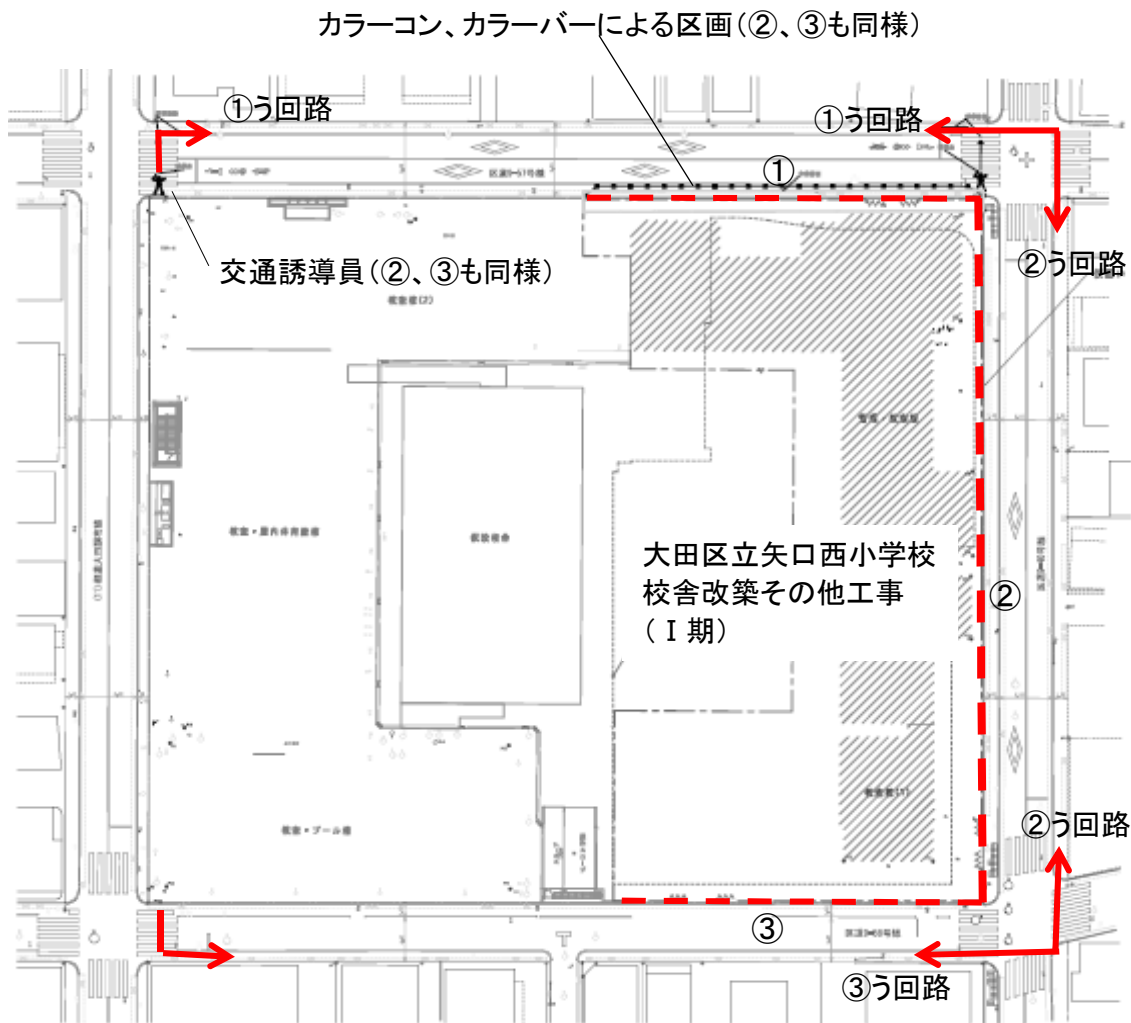
平面図(う回路図)
